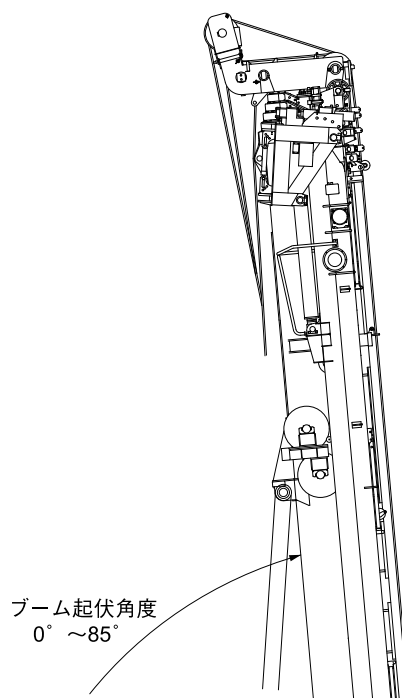
50tonフック
