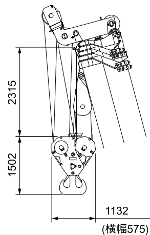
130tonフック
