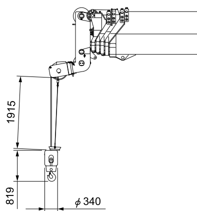
7.8tonフック
