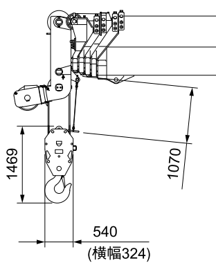
50tonフック
